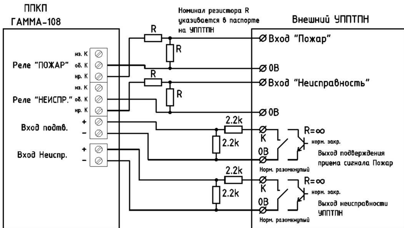
Пример подключения к нормально разомкнутым контактам
